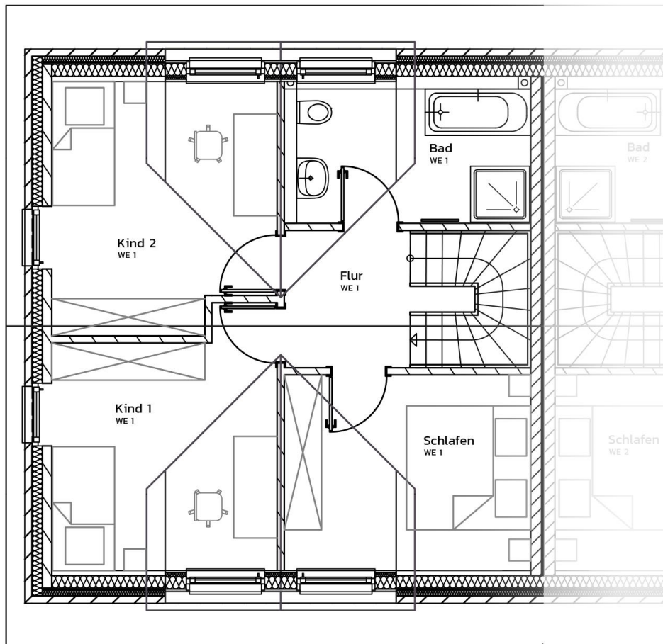
Grundriss DG
