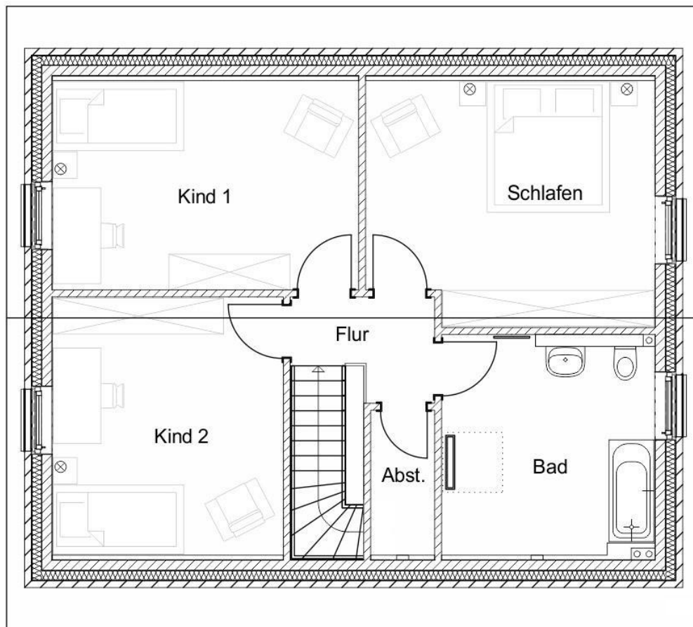
Beispielgrundriss DG
